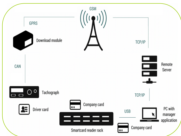
Bloková schéma DigiSafe
